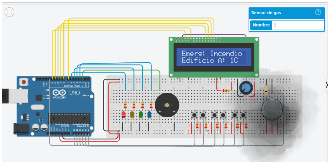
Figura 10 Interfaz del funcionamiento del sensor de MQ-2
