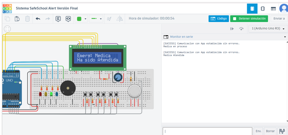
Figura 5 Interfaz del circuito al cambiar el estado de una emergencia a Atendida
