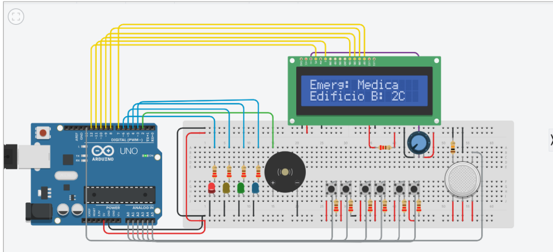
Figura 11 Interfaz de mensajes dinámicos en LCD.
