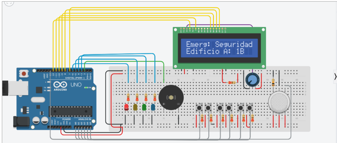
Figura 9 Interfaz de activación sirena de emergencia activa.
