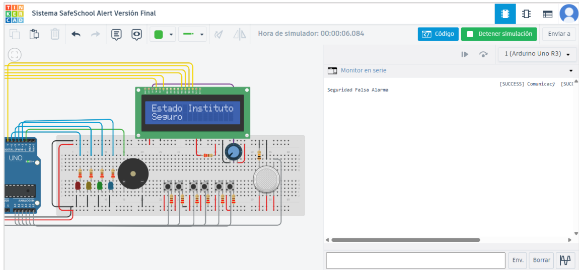
Figura 2 Interfaz del circuito en estado seguro (Sin emergencias).
